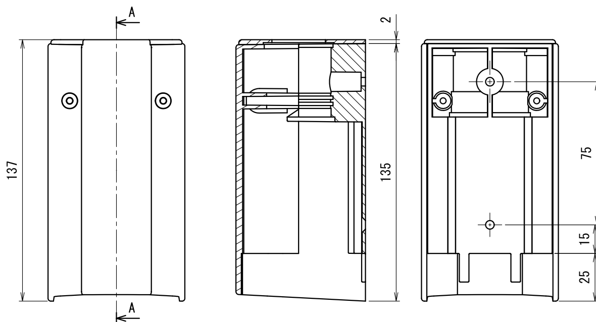
断面 A-A
